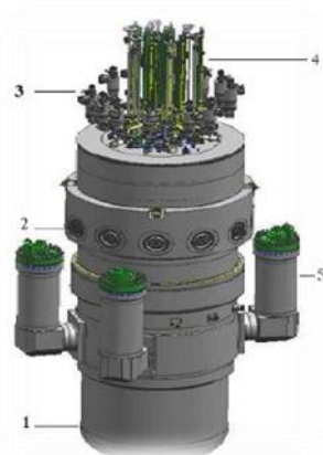
2-rasm. RITM-200H yadro reaktori tuzilishi.
