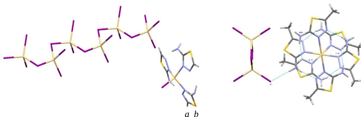
1-расм. [\text{Cd}(\text{atdz})_3\text{I}] \cdot [\text{CdI}_3] (a) ва [\text{Cd}(\text{matdz})_6] \cdot [\text{Cd}_2\text{I}_6] (b) комплексларининг кристалл тузилишлари.
