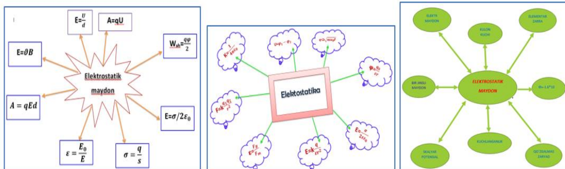
1-rasm. Fizik kattaliklarning KLASTERI
