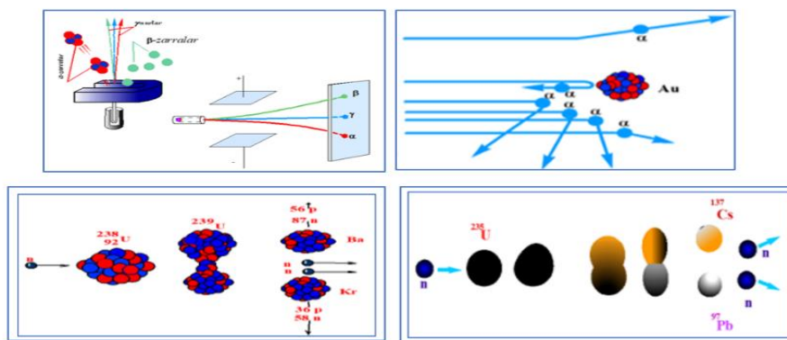
Tabiiy radioaktivlik hodisalaridan namunalar.
