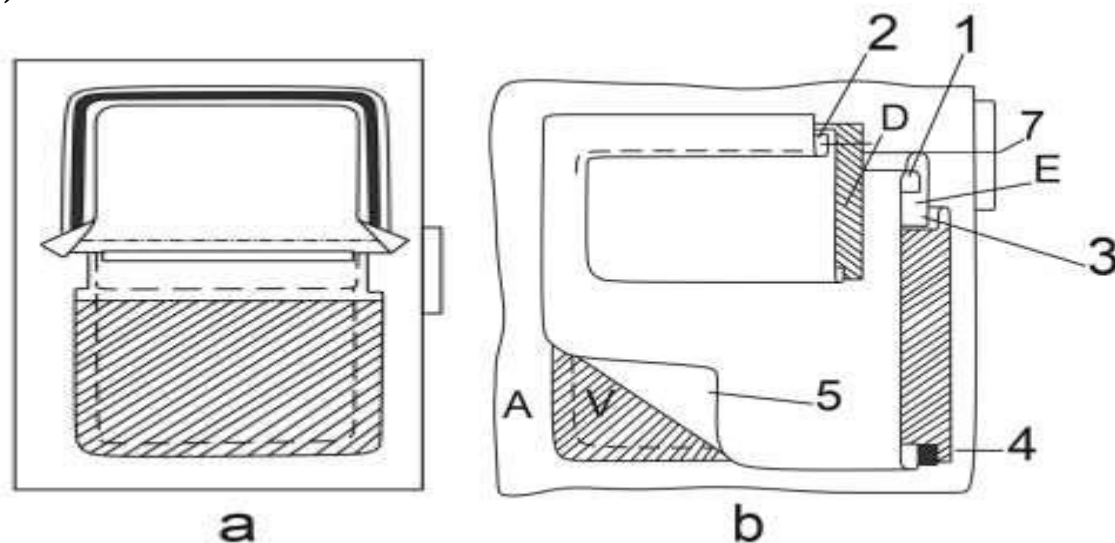
3-rasm. Qoplama cho'ntakni old bo'lakka yelimlab yopishtirish
