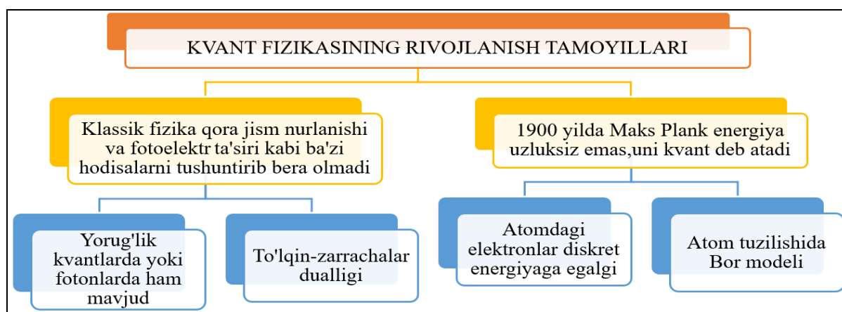
1-rasm. Kvant fizikasining rivojlanish tamoyillari.
