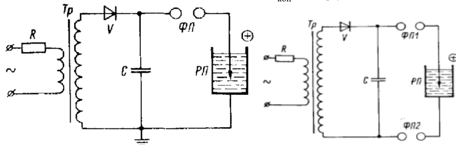
Рис.1 Электрическая схема для воспроизведения ЭГЭ а) с одним формирующим промежутком б) с двумя формирующими промежутками
