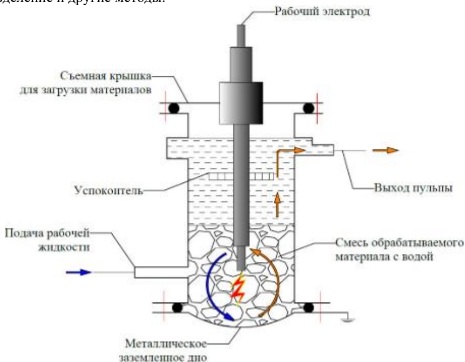
Рис.2. Конструктивная схема и принцип организации процесса удаления от глины твердых фракций руды в рабочей емкости электрогидравлической установки
