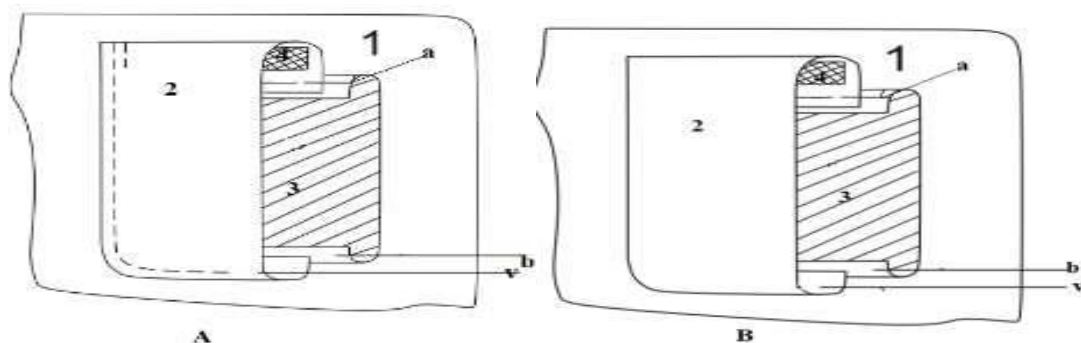
2-rasm Astarli qoplama cho'ntakni old bo'lakka biriktirish
